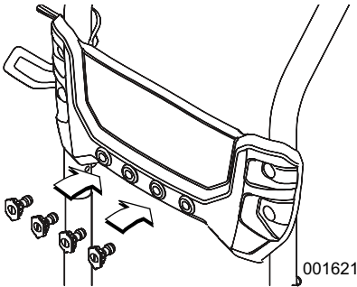
Figura 2-3. Inserción de las boquillas
