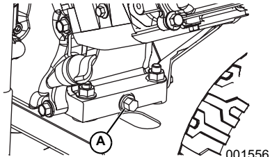
Figure 4-7. Bouchon de vidange de l'huile
