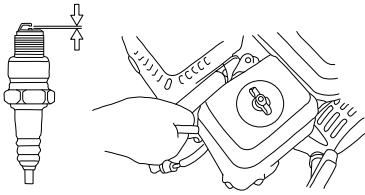
Figure 4-8. Bougie d'allumage
